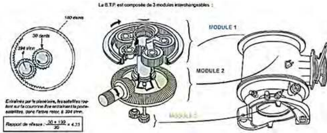
Figure 141 - Boîte de transmission principale épicycloïdale
