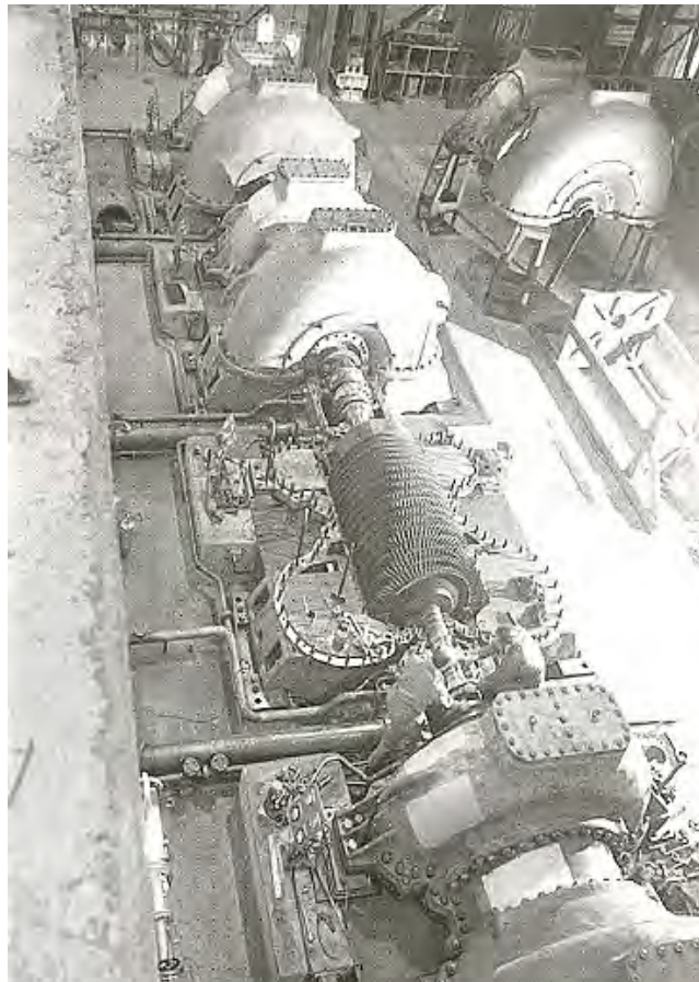
Fig. 8 Compresseur TB (Rateau) en cours de maintenance
