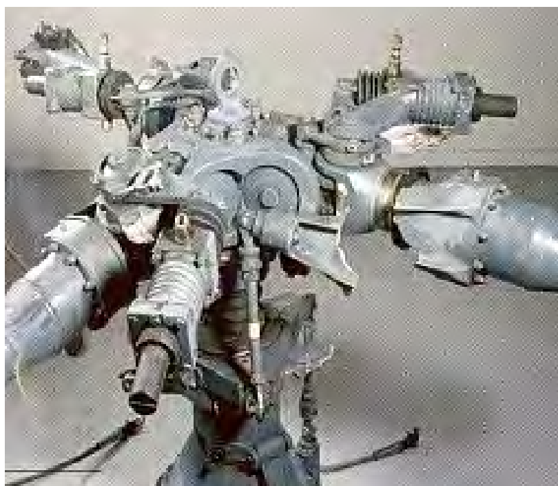
Fig. 26 Tête de rotor d'hélicoptère en expertise
